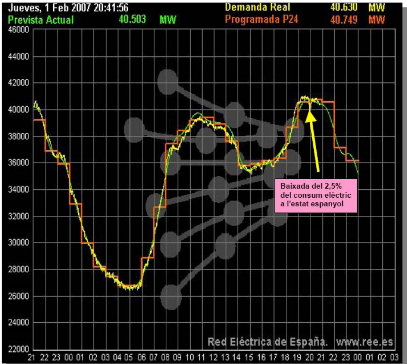
Gràfic de la demanda real en la Xarxa Elèctrica espanyola de l'anterior convocatòria de febrer de 2007
